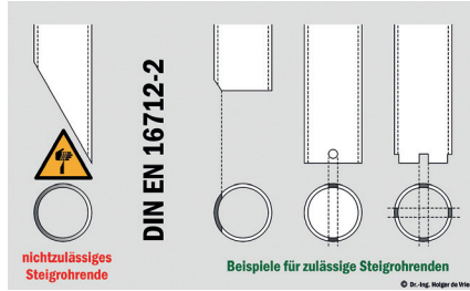
Abbildung 14: Nichtzulässige und zulässige Steigrohrenden für Ansaugschläuche nach DIN EN 16712-2
