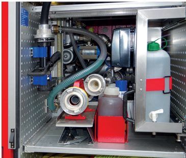
Abbildung 15: TLF 3000 mit festeingebautem Schaummittelbehälter und „Zapfstelle“ im Geräteraum G4
