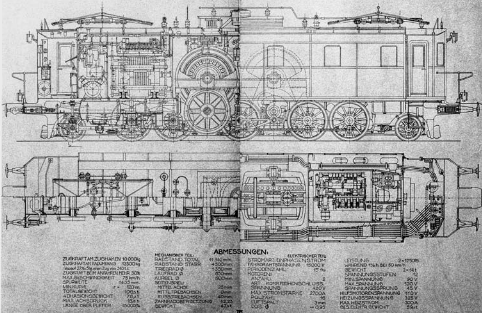
1-E-1 ÖERLIKON-LOKOMOTIVE FÜR DIE LOTSCHBERGBAHN
