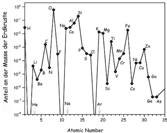
Abb. 1.3 Die Liste der Zutaten für erdähnliche Planeten. Dargestellt ist die relative Häufigkeit der Elemente in der Erdkruste. Man beachte,
