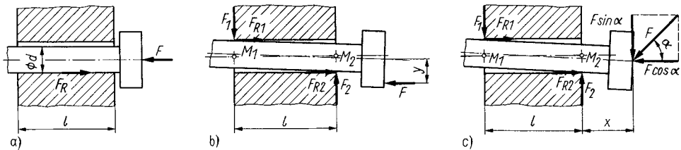
Bild 9.1 Kraftangriff bei Gleitführungen
