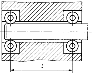
Bild 9.9 Prinzip einer Rollenführung
