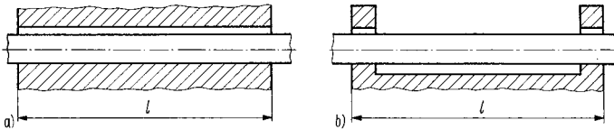
Bild 9.2 Gleitführungen a) einstellig; b) zweistellig
