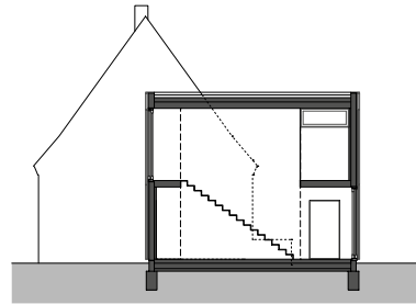
Schnitt
