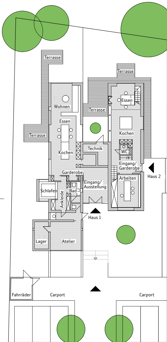
Erdgeschoss
